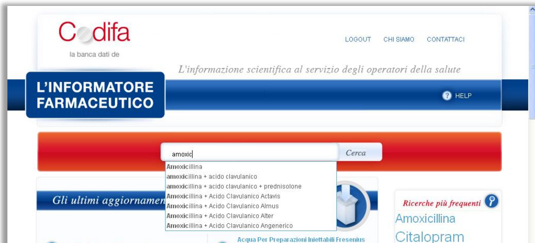
Figura 8 - Ricerca assistita
